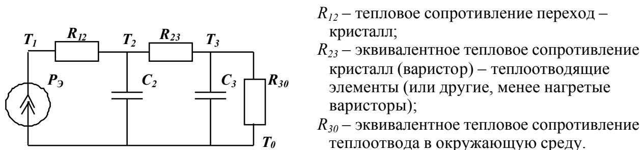
Рис. 1. Упрощенная термическая модель ОПН
